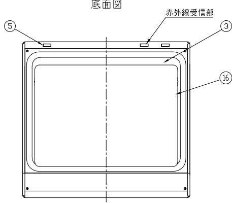
底面図
