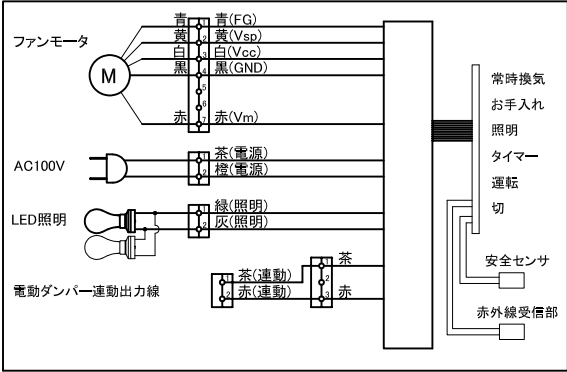
□結線図
