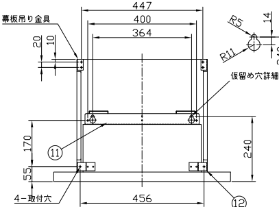
背面取付図
