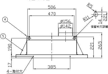
背面取付図
