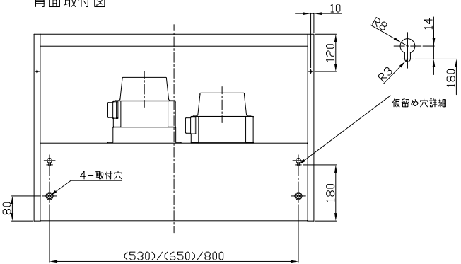
背面取付図
