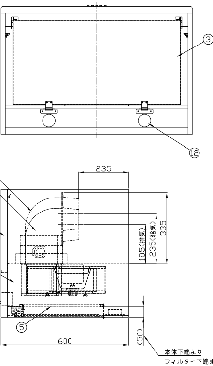
底面図
