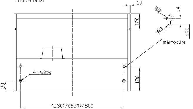
背面取付図
