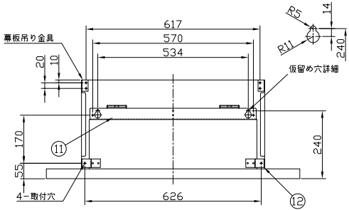
背面取付図
