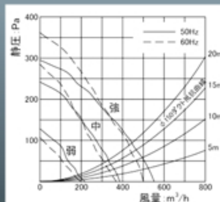
静圧・風量曲線
