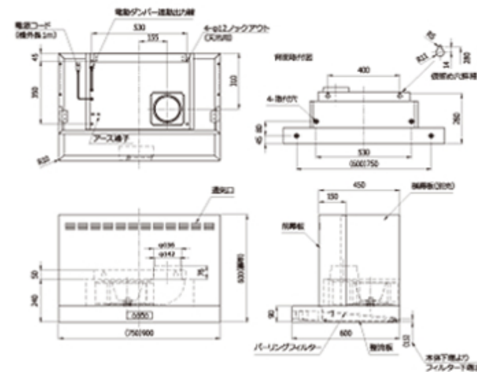
製品寸法図
