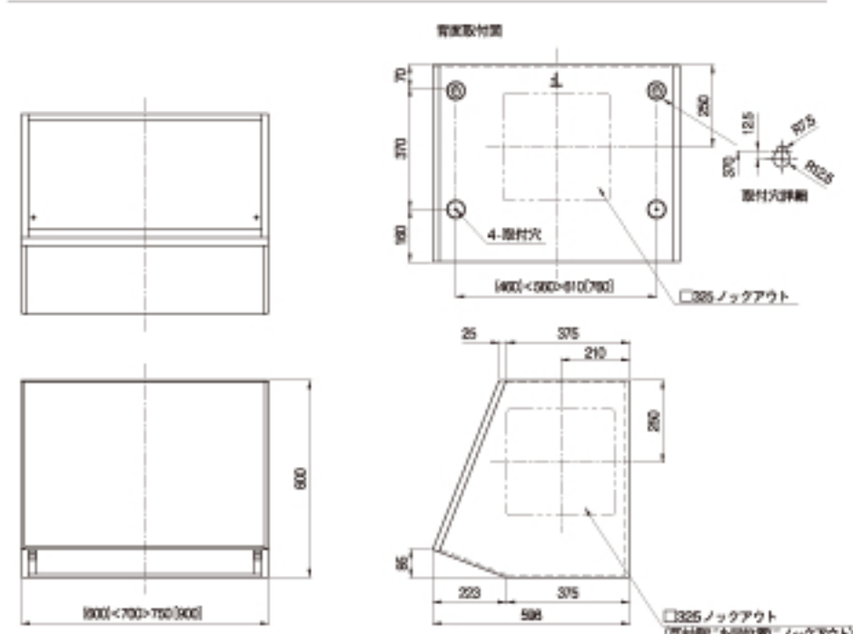
製品寸法図
