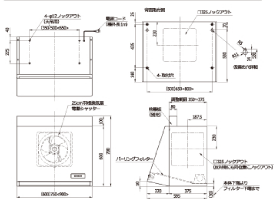
換気扇単品寸法図
