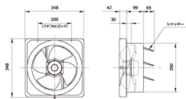
換気扇単品寸法図
