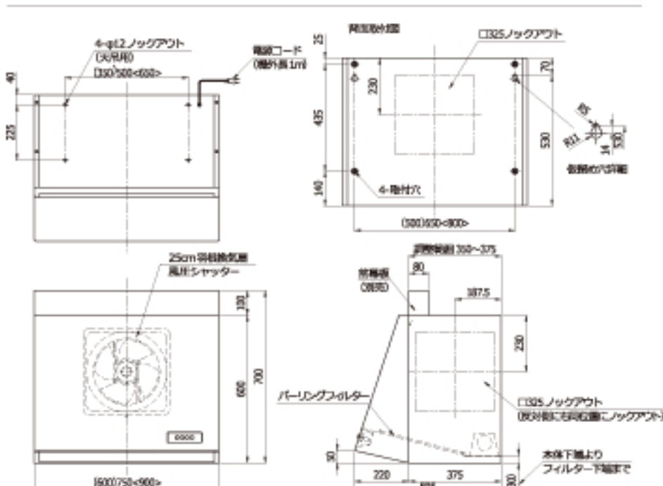
製品寸法図
