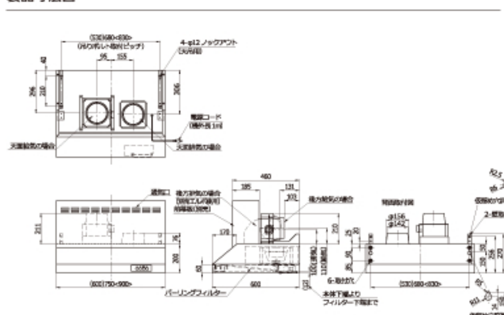
製品寸法図
