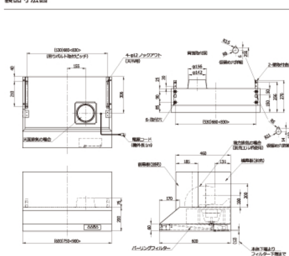
製品寸法図
