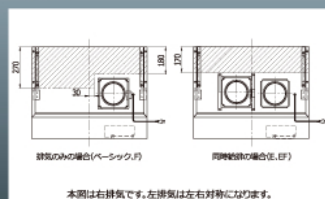
梁対応図
